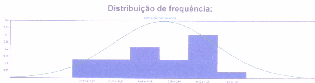
Figura 58 - Distribuição de Frequência.
