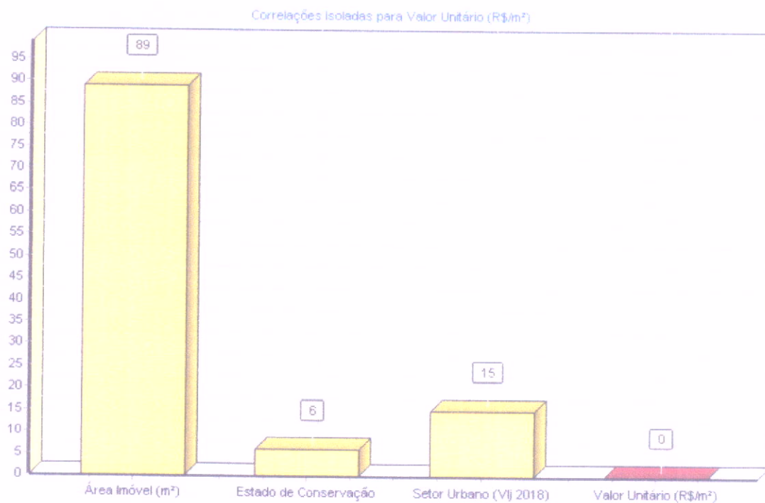
Figura 16 - Correlações Isoladas para Valor Unitário (R$/m²).
