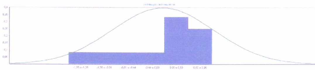
Figura 25 - Distribuição de Frequência.
