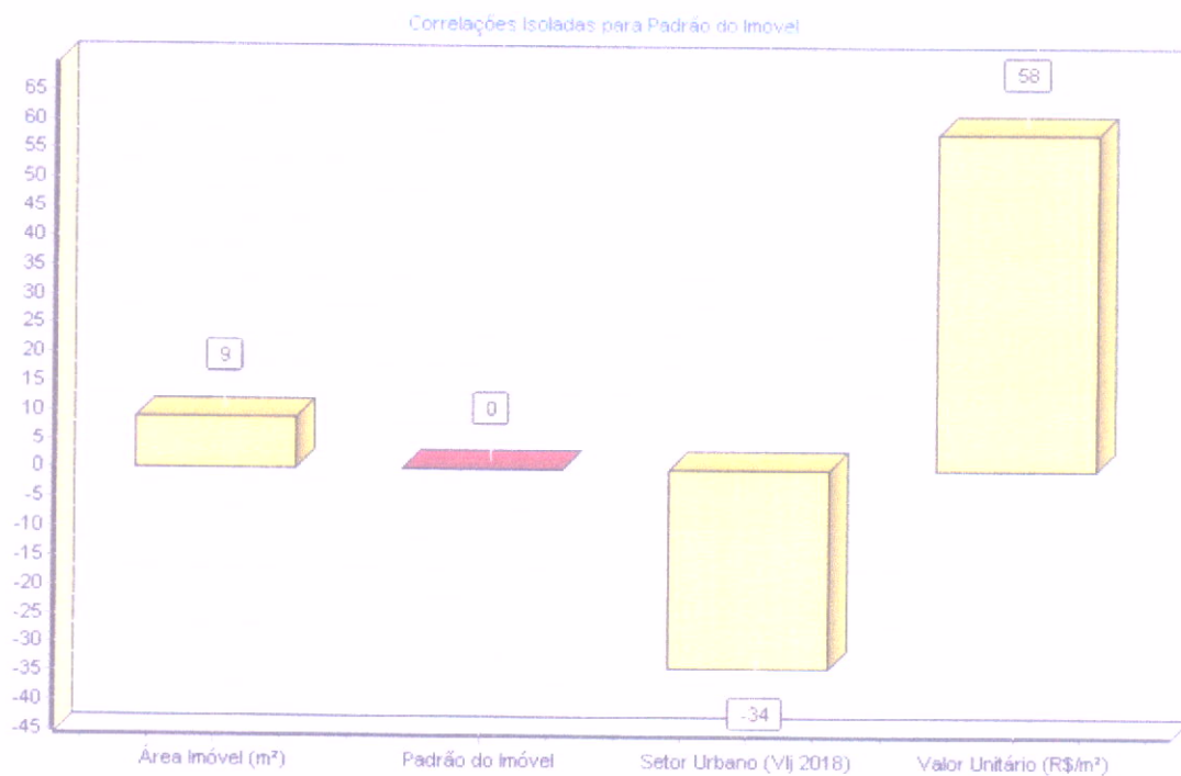
Figura 45 - Correlações Isoladas para Padrão do Imóvel.
