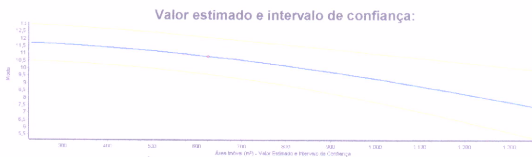
Figura 59 - Área Imóvel (m²) - Valor Estimado e Intervalo de Confiança.
